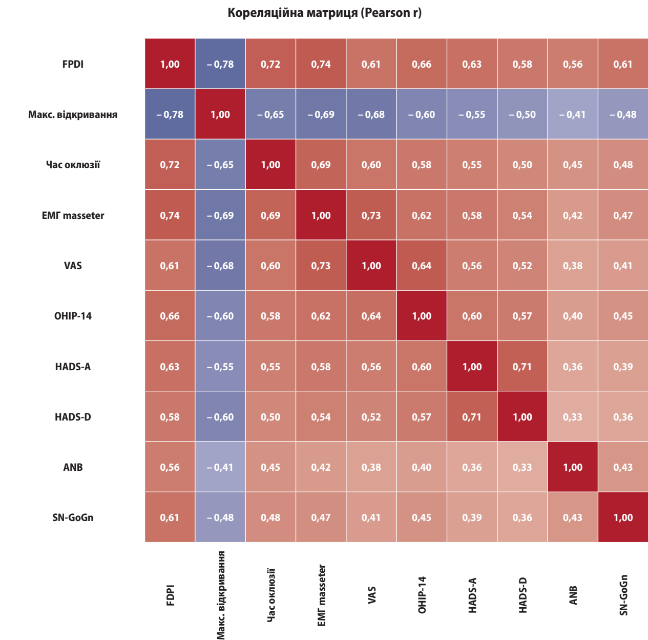
Рис. 2. Кореляційна теплова карта взаємозв'язків між індексом функціональної дезорганізації (FPDI), клінічними, функціональними, електроміографічними, психоемоційними та цефалометричними показниками.
